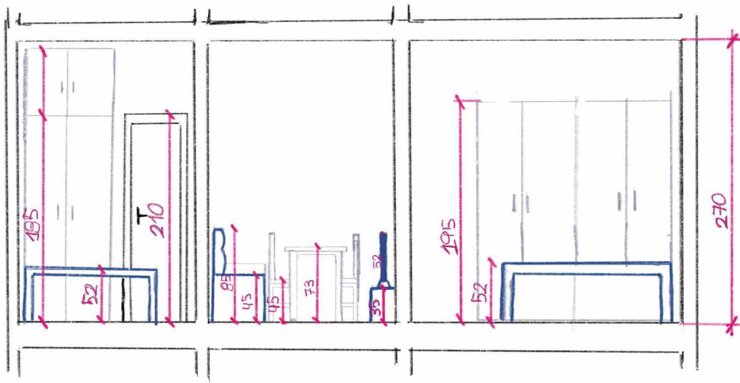
Sección CC'
