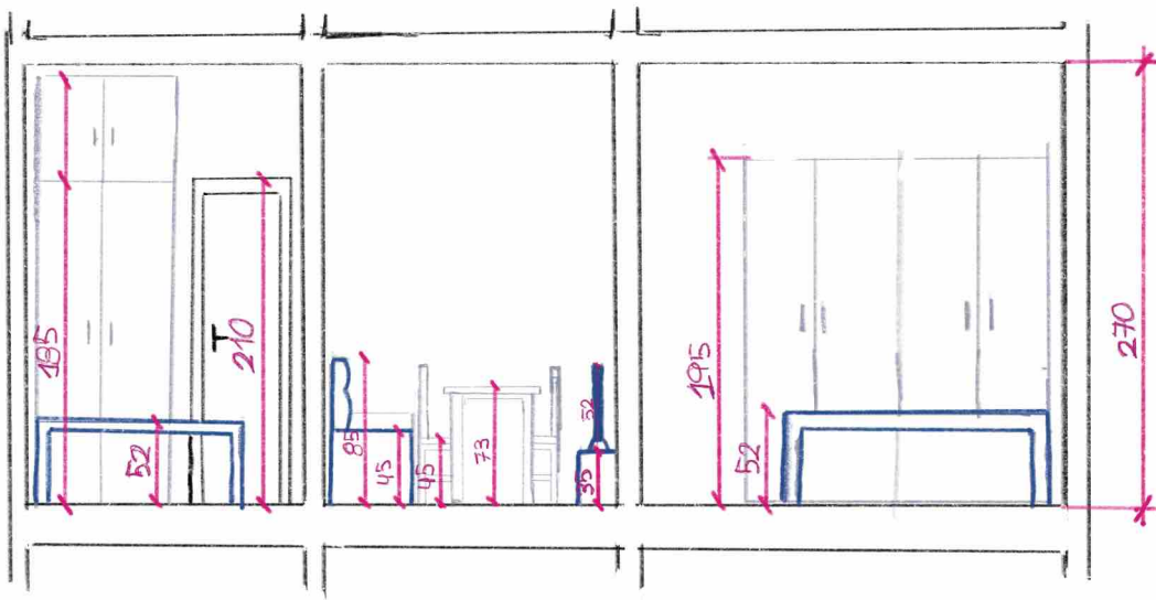
Sección CC'
