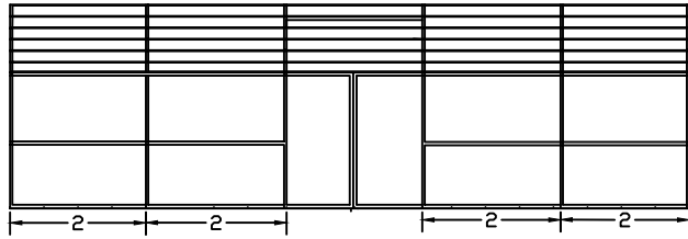
ALZADO
