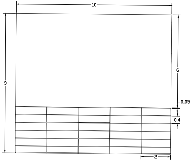
PLANTA SUPERIOR
