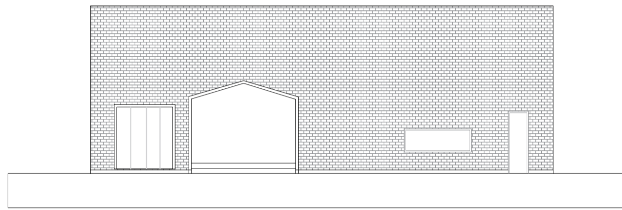
ALZADO NORTE
