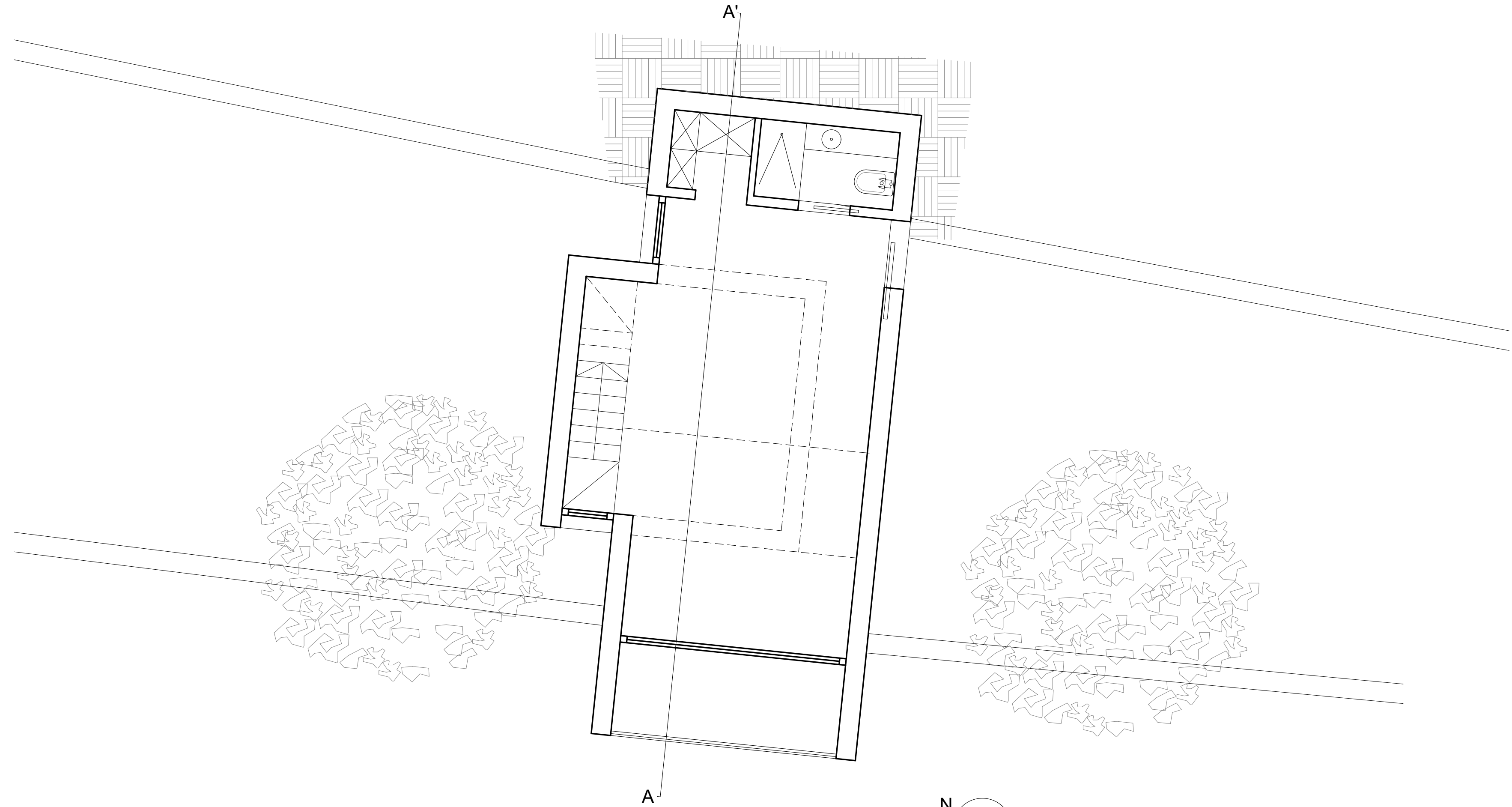
PLANTA BAJA
