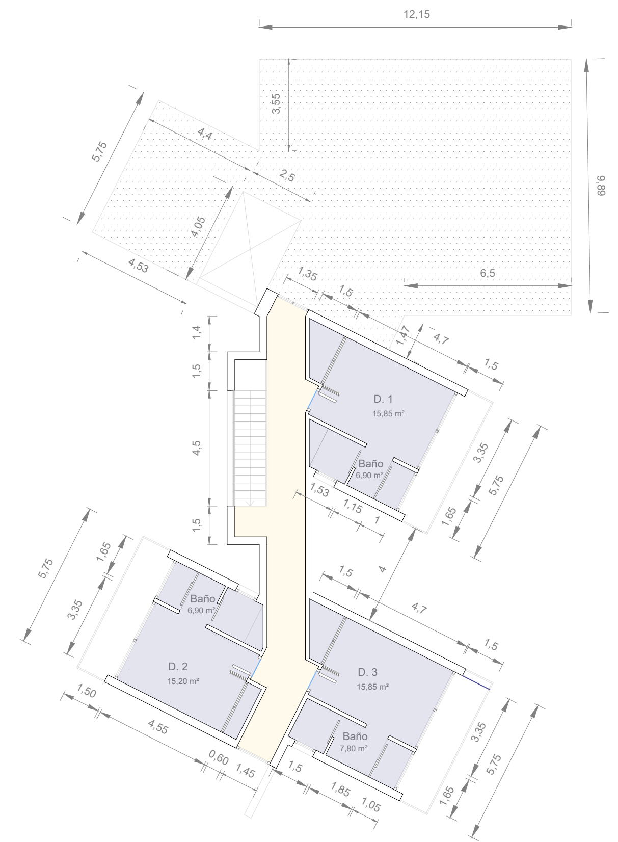
Planta Primera Cota +3,00
