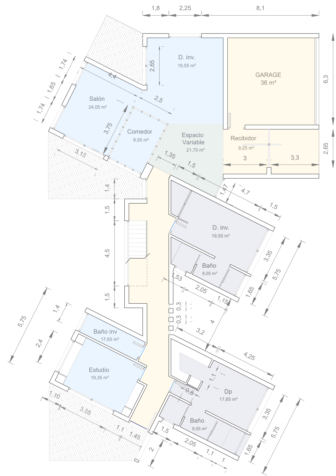
Planta Baja Cota +0,00
