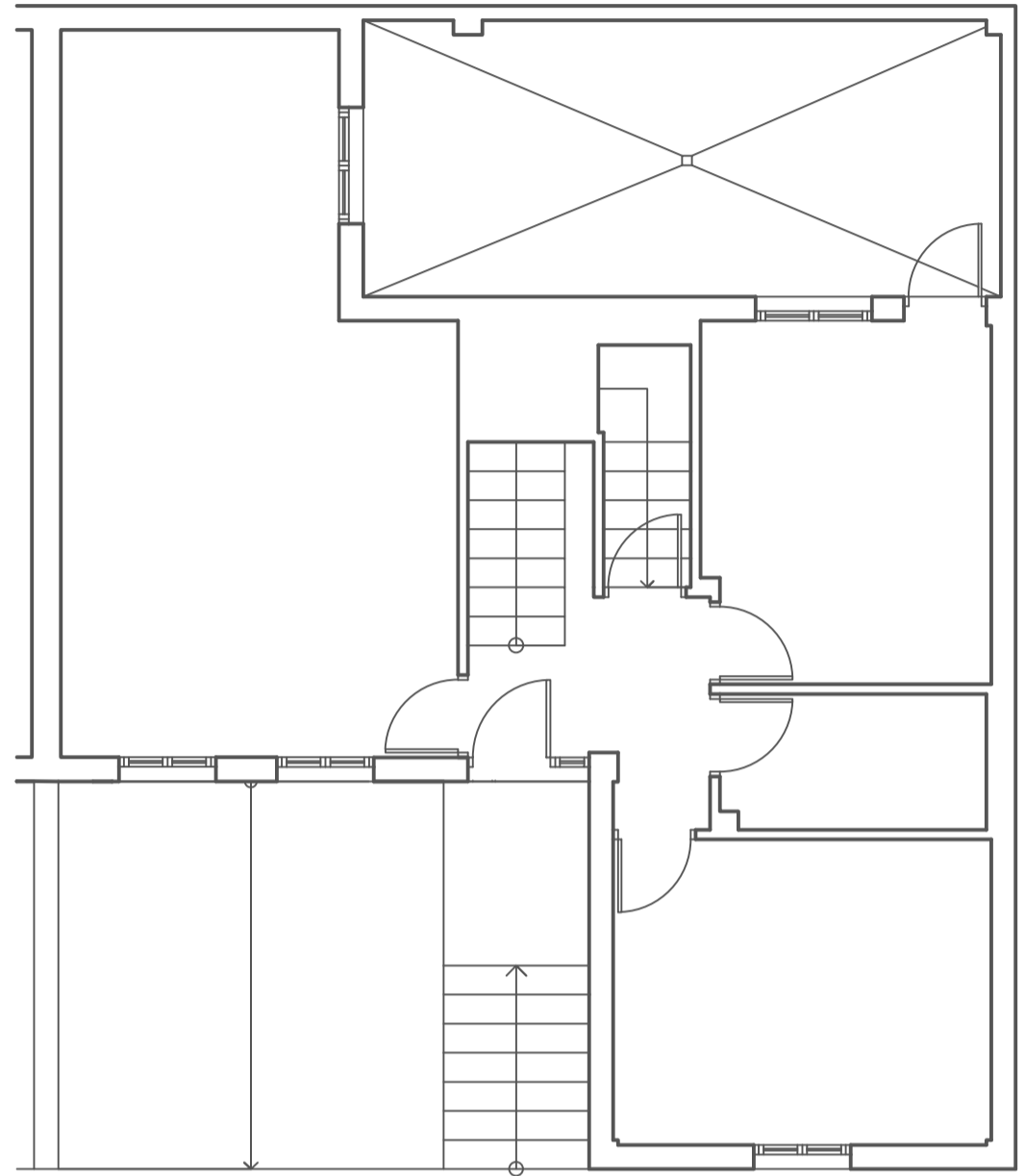
PLANTA MEDIA
