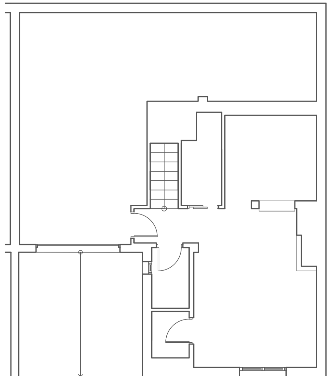
PLANTA BAJA
