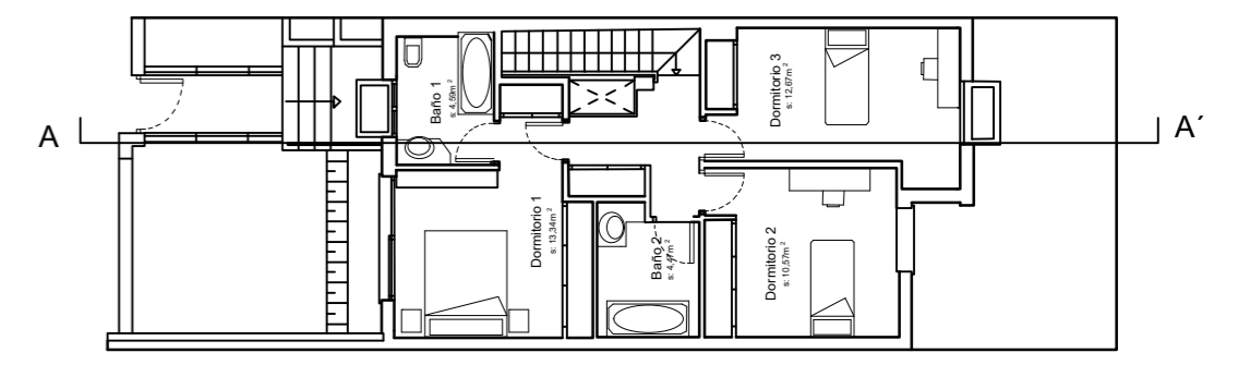
Planta alta
