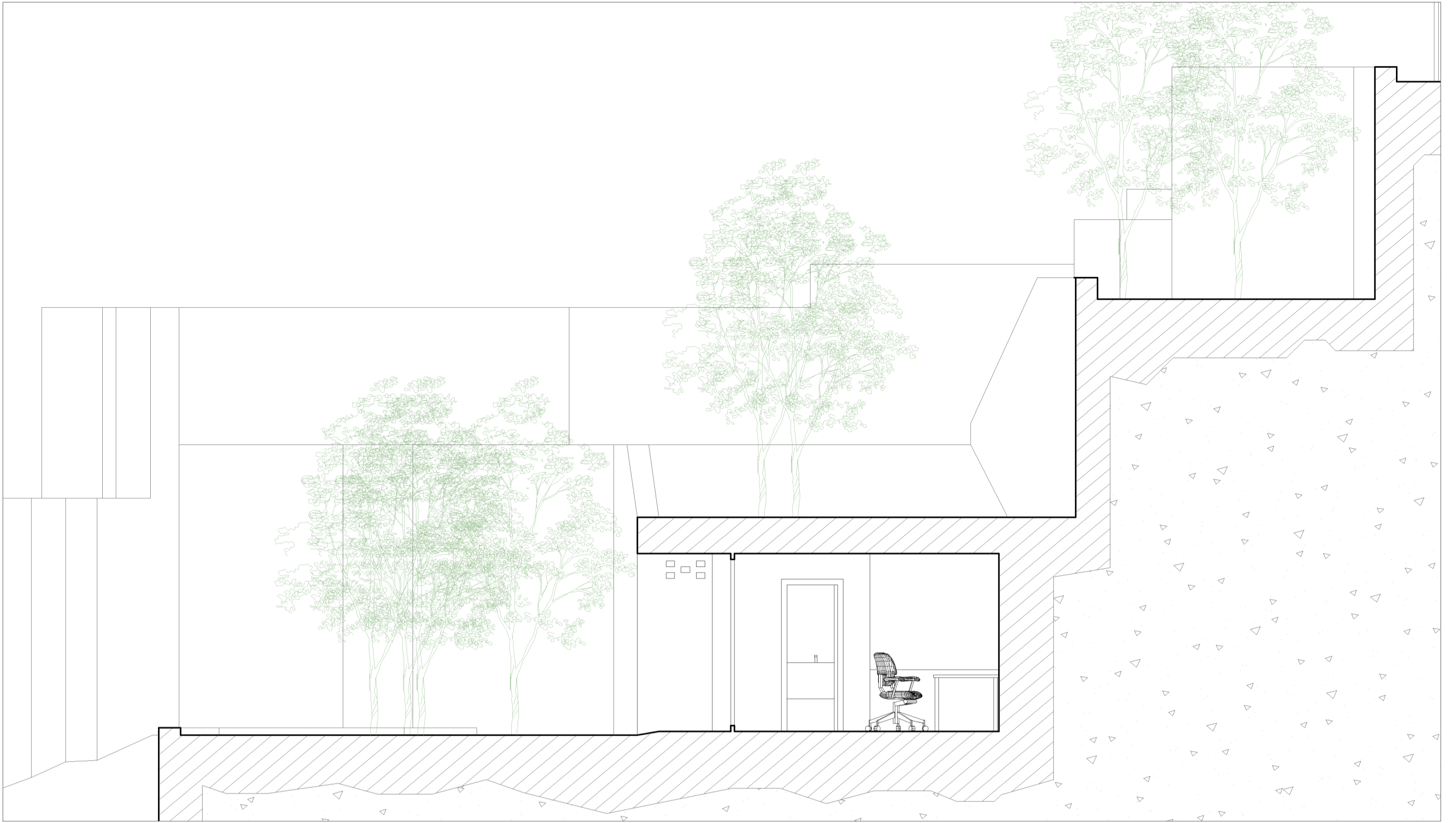
SECCION C-C'
