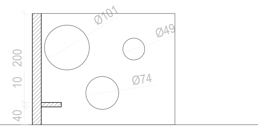
SECCIÓN B·B'
