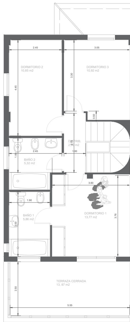
PLANTA ALTA
