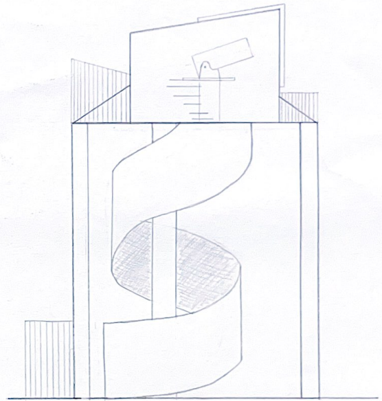
SECCIÓN MIRADOR
