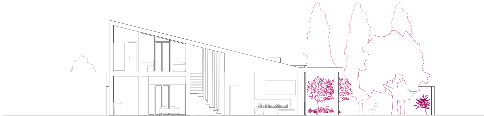
SECCIÓN B-B'
