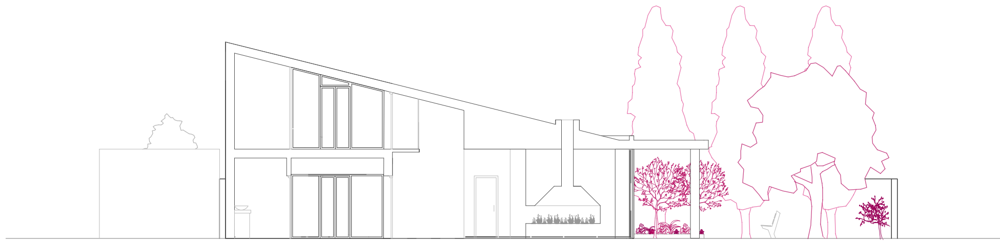
SECCIÓN A-A'
