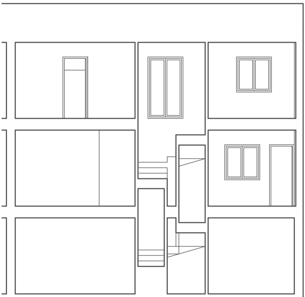
SECCION C-D
