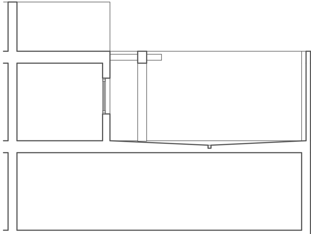
SECCION A-B
