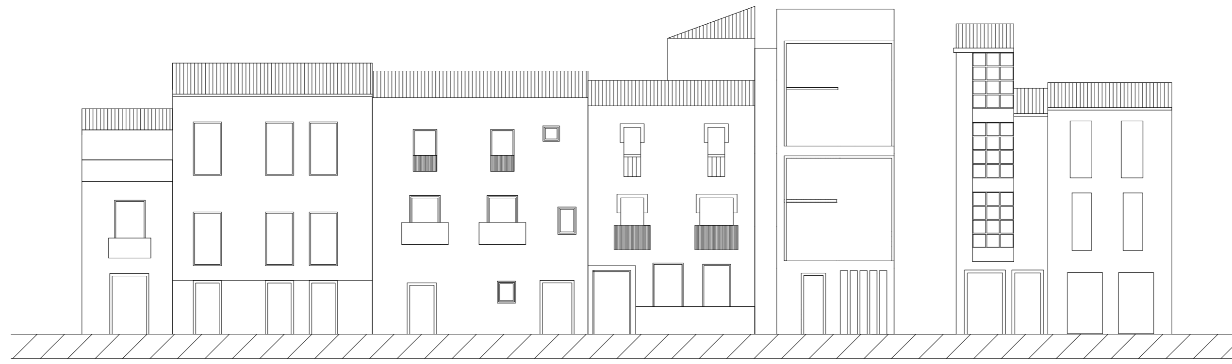
ALZADO CALLE MOLINOS
