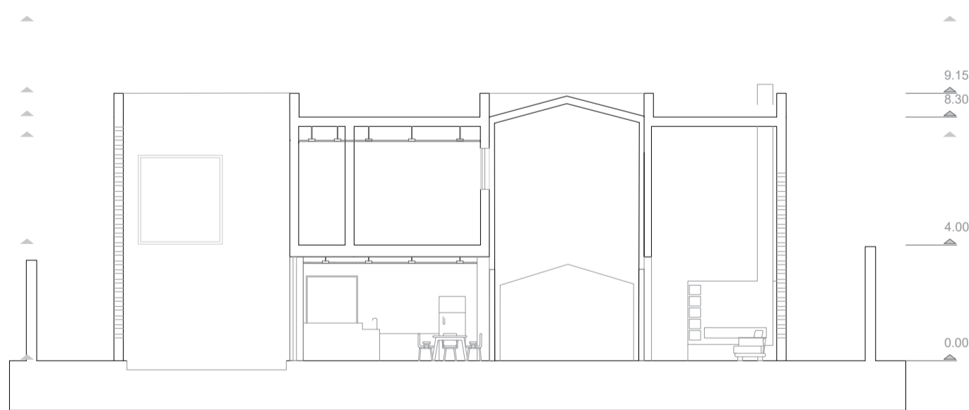
SECCION B B'
