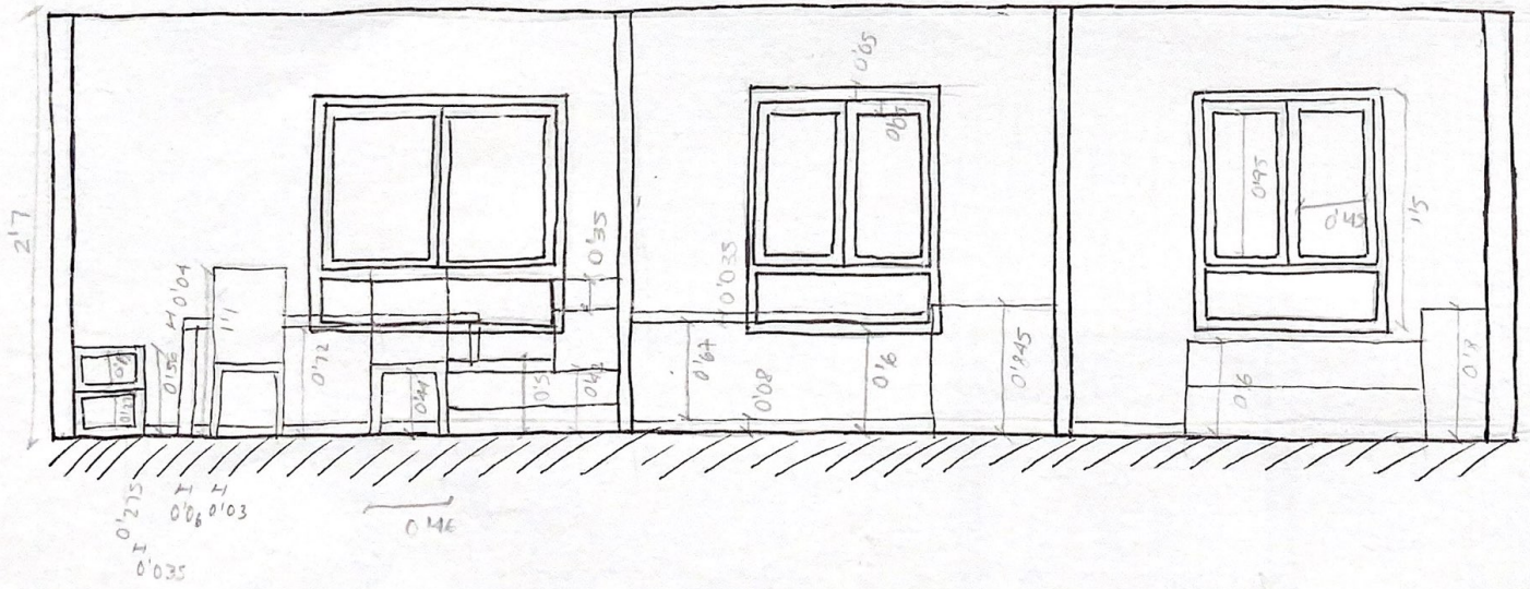
SECCION E-E
