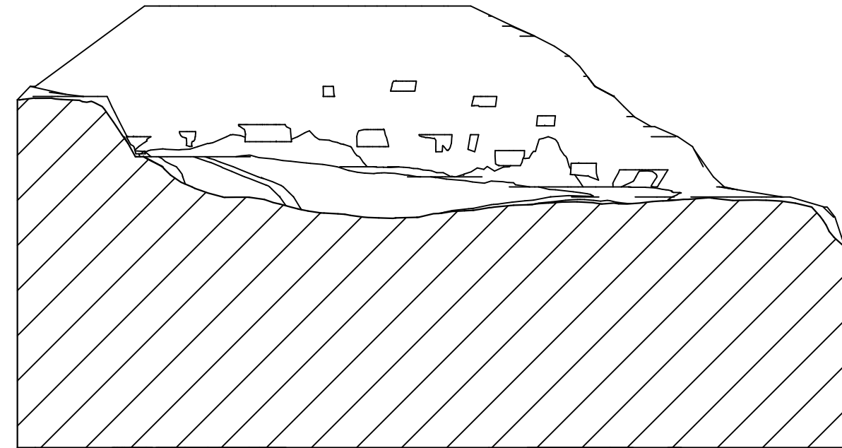
Sección CC'
