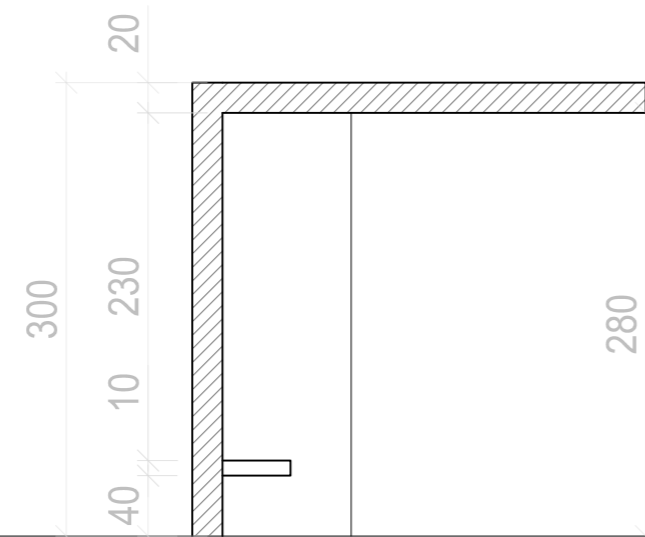
SECCIÓN A-A'
