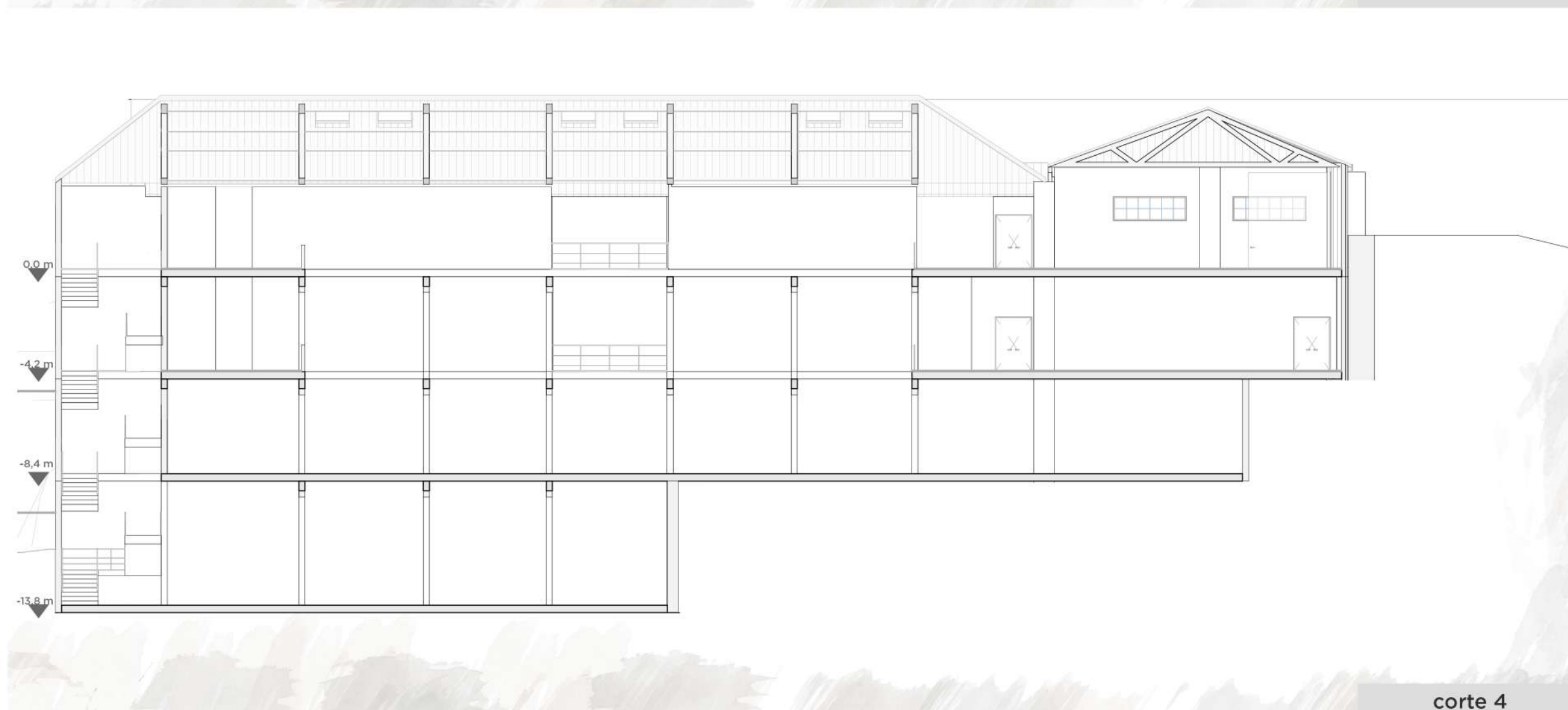
corte 4
