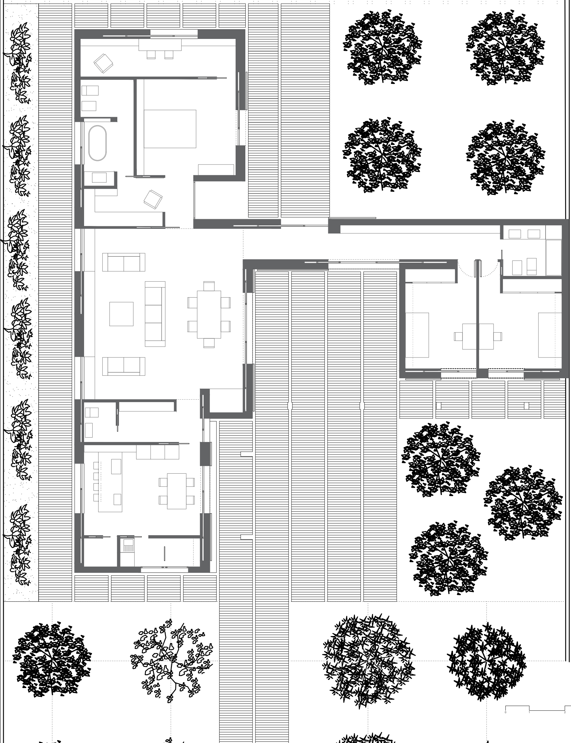
PLANTA CON EXTERIOR ESCALA 1/100
