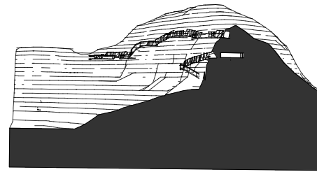
SECCION B-B'
