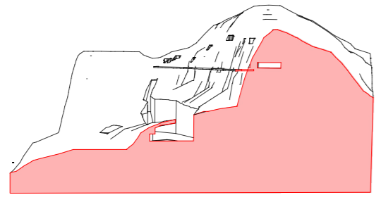
SECCION E-E'
