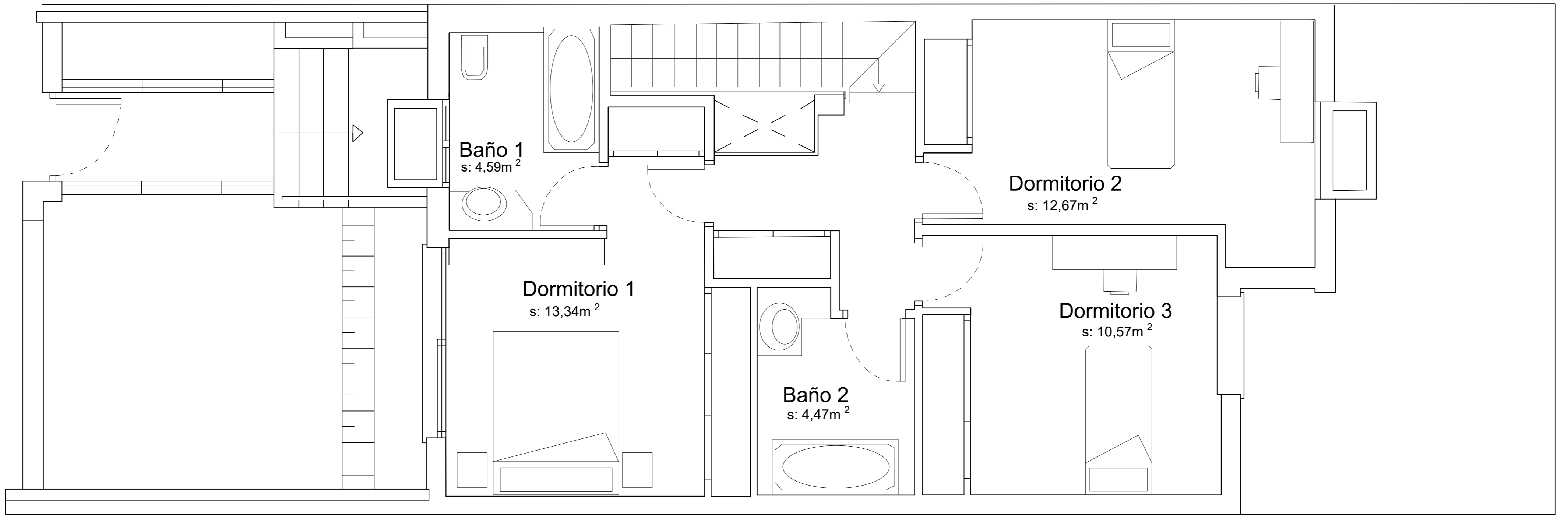
Planta alta
