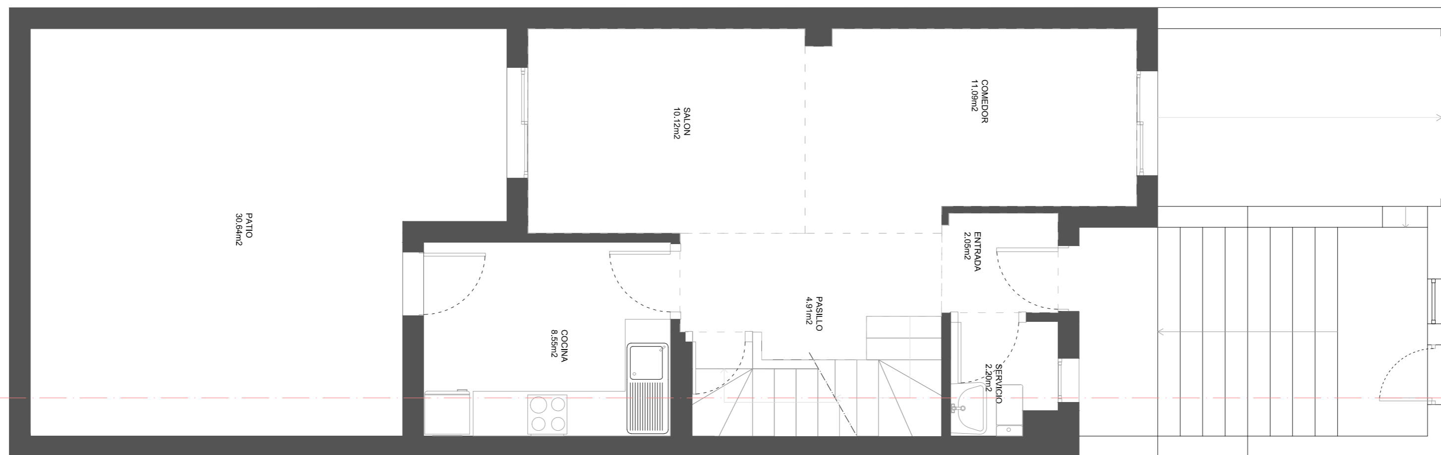
PLANTA PRIMERA
