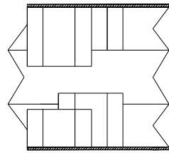
Sección C'-C
