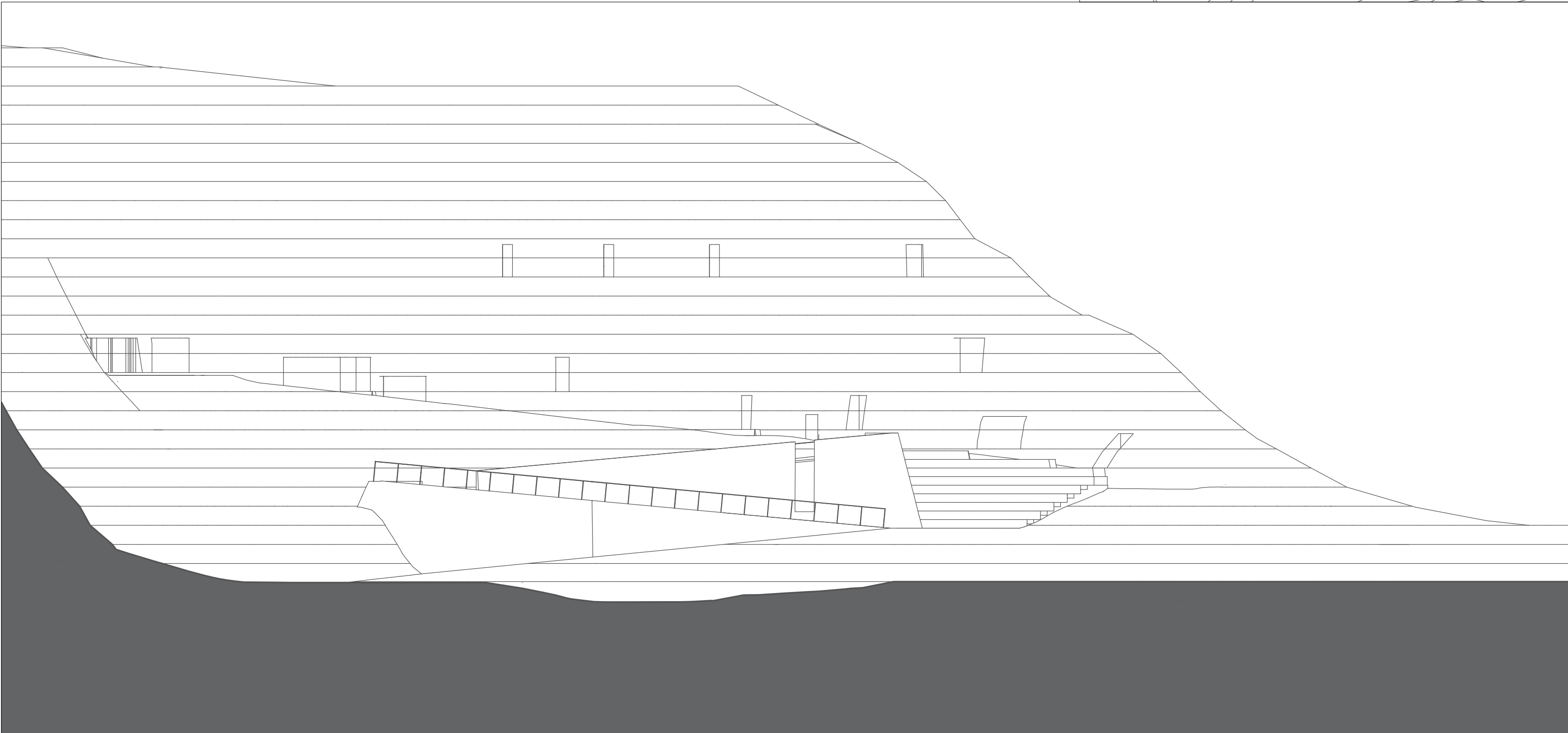
SECCIÓN FRONTAL 1
