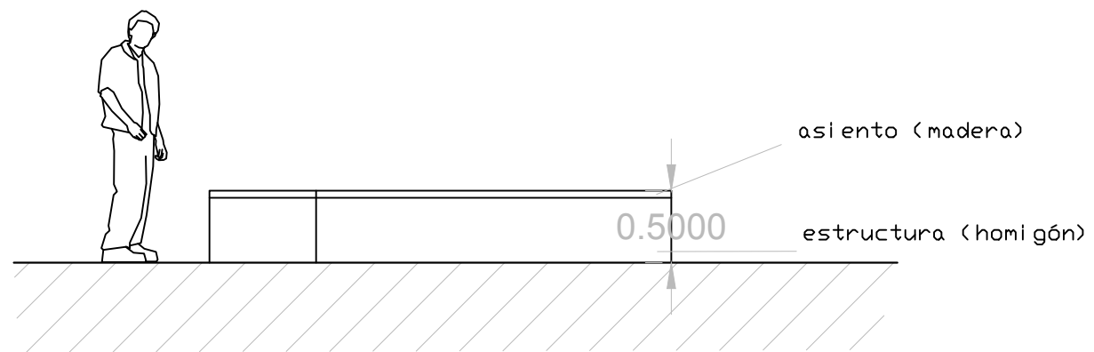
ALZADO-SECCIÓN
