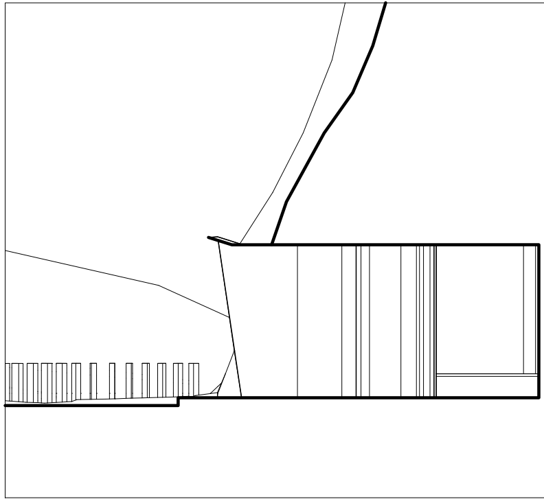
SECCIÓN 1-1' CUEVA 1
