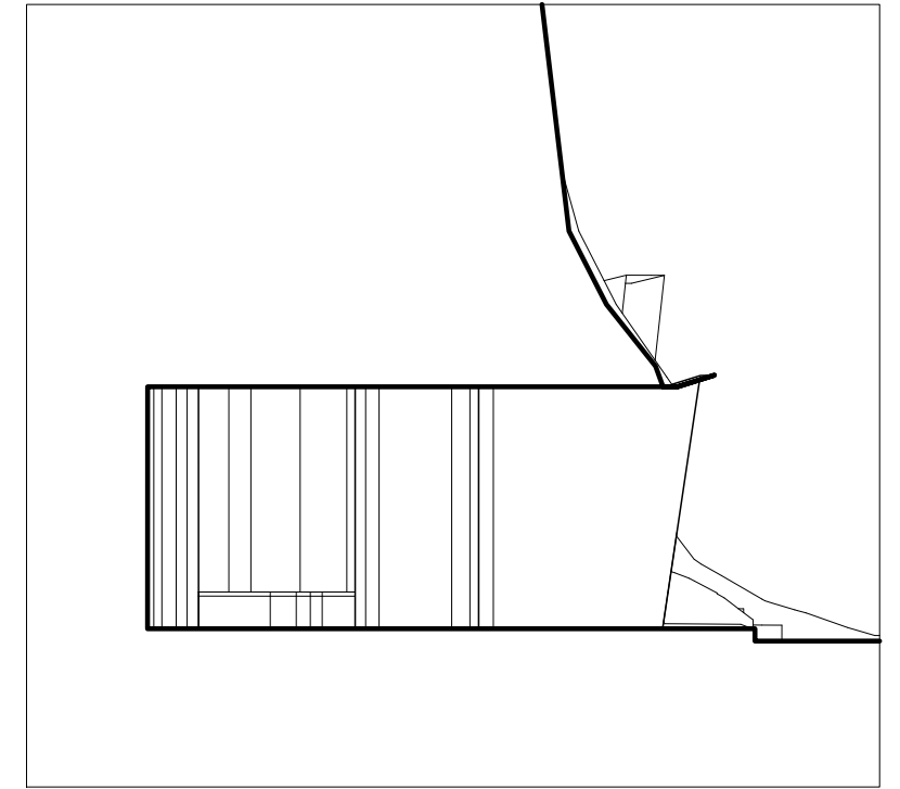
SECCIÓN 1-1' CUEVA 1
