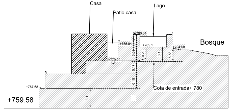
Seccion Transversal
