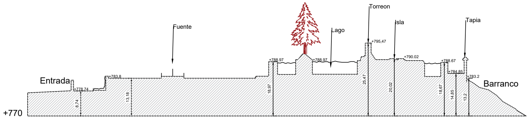
Seccion Longitudinal
