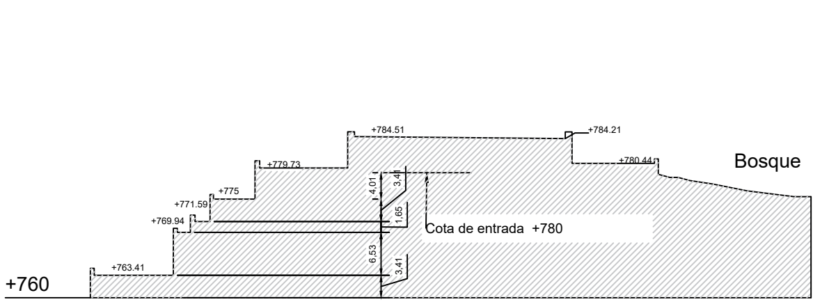
Seccion Transversal
