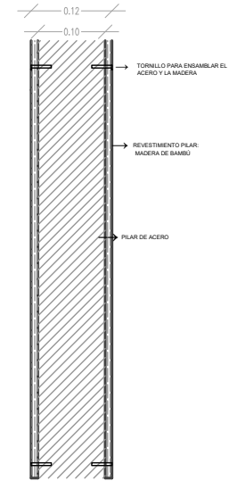
DETALLE DEL PILAR DE ACERO REVESTIDO DE MADERA Y ENSAMBLADO CON TORNILLOS
