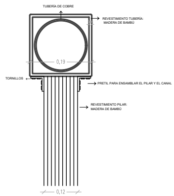
DETALLE DEL ENSAMBLAJE DEL PILAR Y EL CANAL
