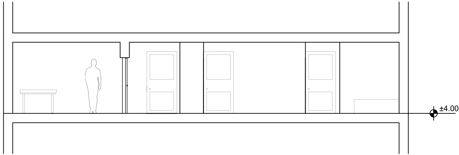
Sección AA'
