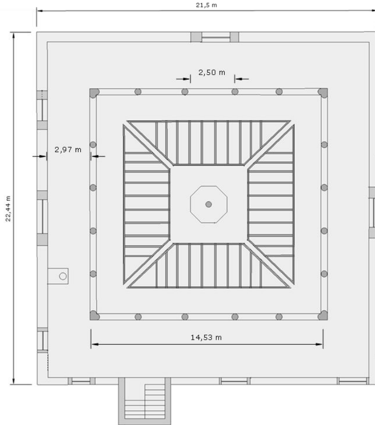
PLANTA BAJA SIN HABILITAR
