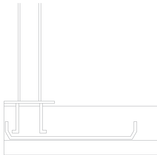
DETALLE ENCUESTRO PILAR-PLATAFORMA
